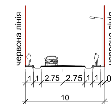
Профіль 2 - 2
