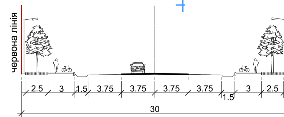
Профіль 1 - 1
